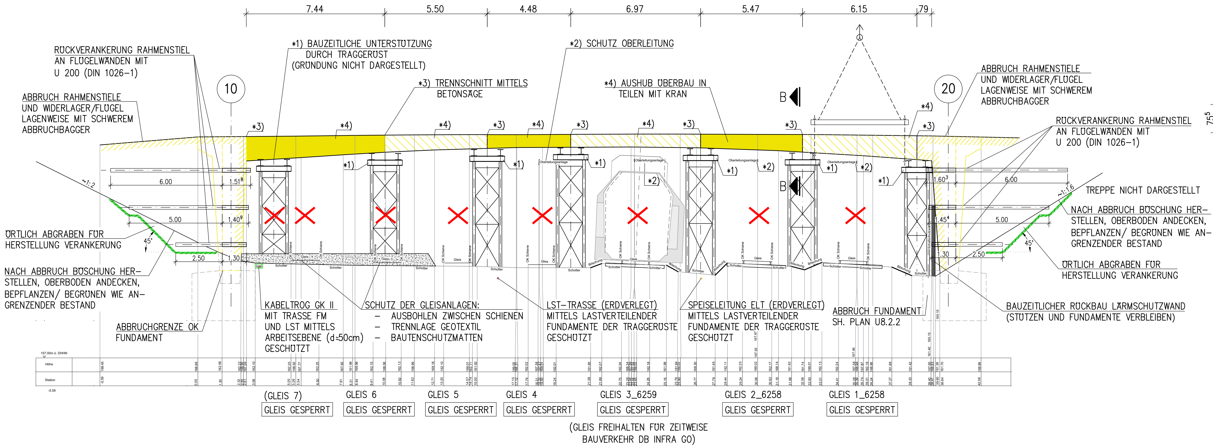
ANSICHT A-A M 1:100
